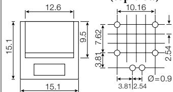
PCBレイアウト
