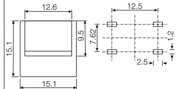
PCBレイアウト
